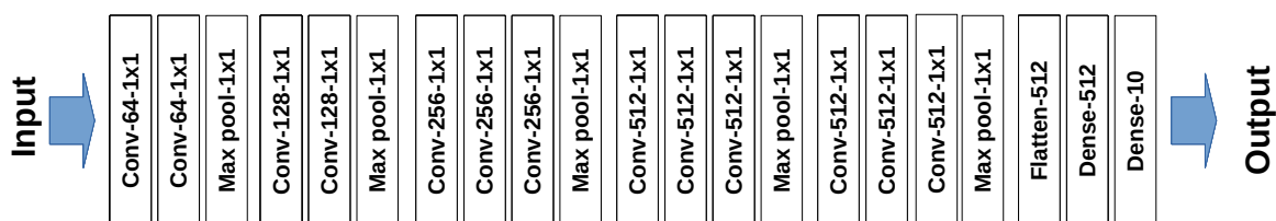
Figura 4.3: Estructura del modelo VGG16. Todas las capas contienen una activación ReLU, excepto la última que contiene un softmax para la clasificación.
