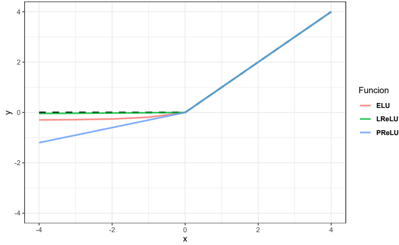
Figura 2.3: Ejemplos de ReLU y algunas de sus variantes. La línea trazada representa el ReLU base. El parámetro para PReLU y ELU es \alpha = 0.3
