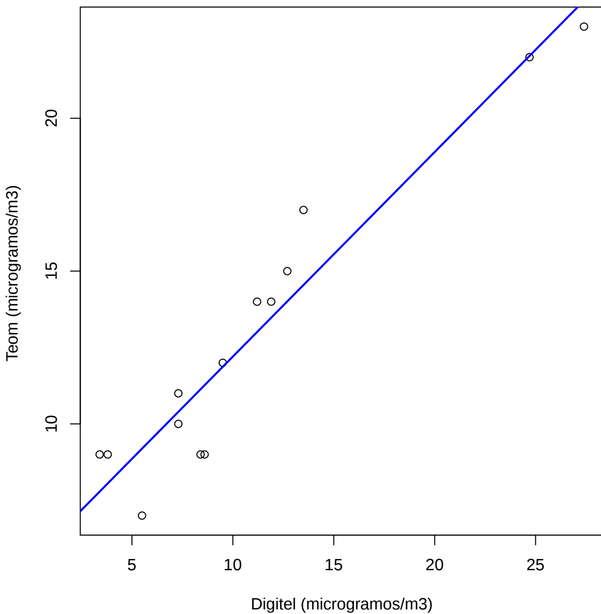
Modelo de regresión lineal
