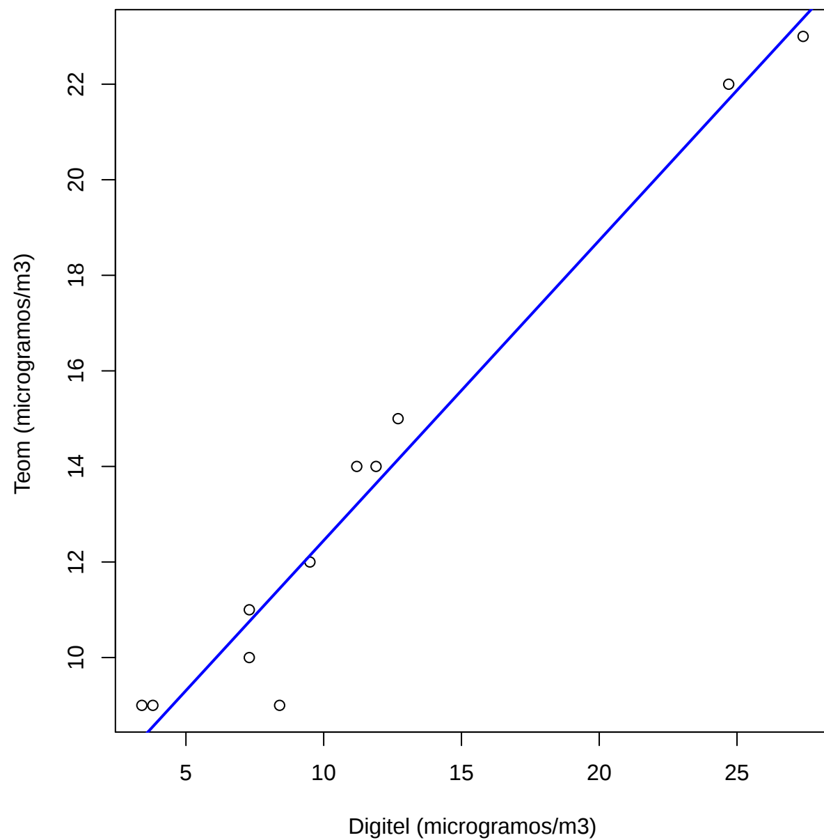
Modelo de regresión lineal sin outliers
