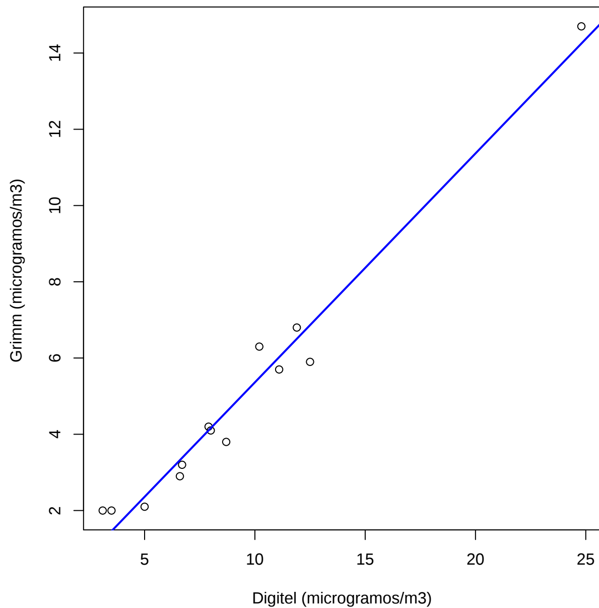
Modelo de regresión lineal sin outliers
