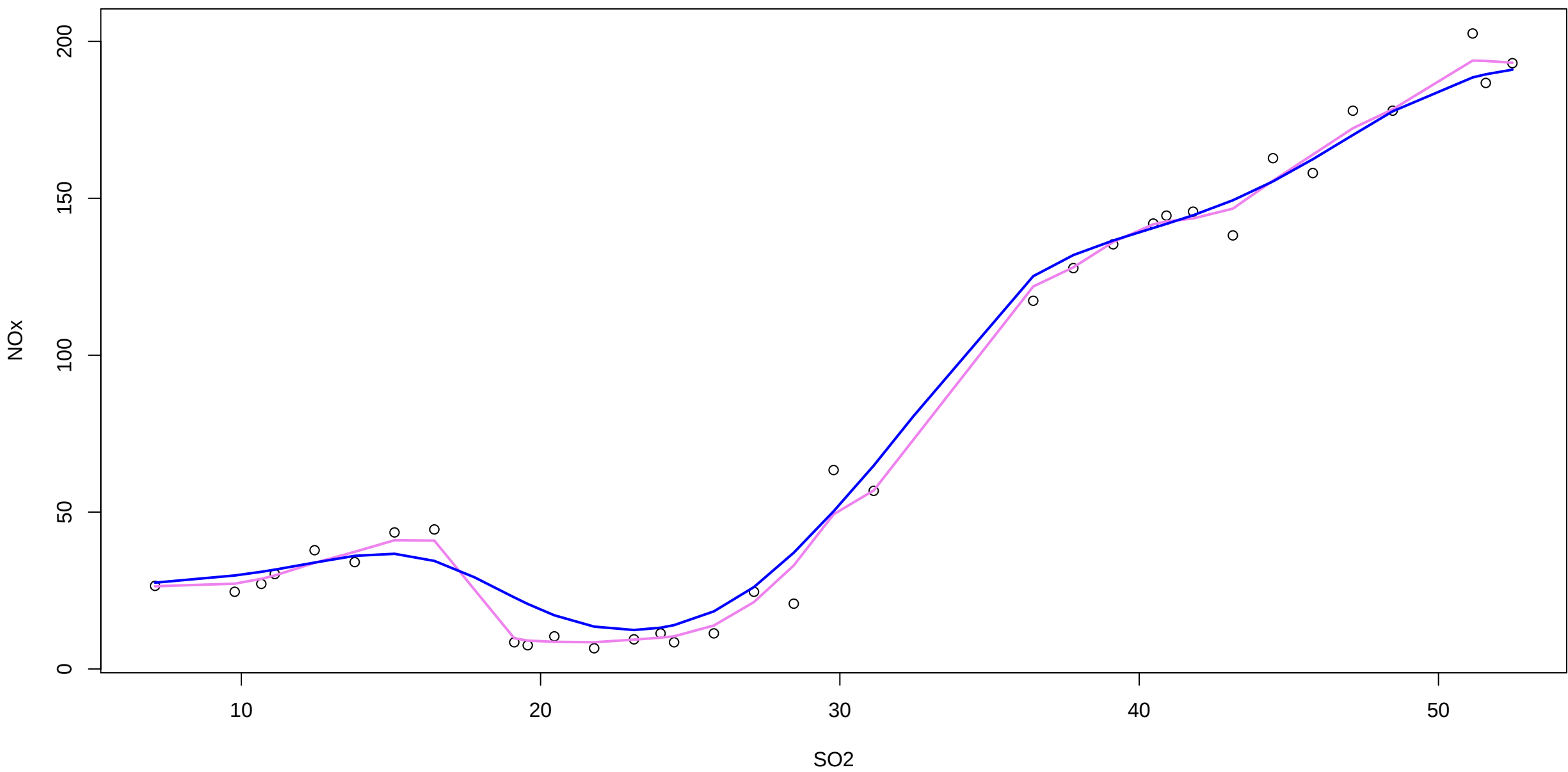
Estimador Nadaraya-Watson
