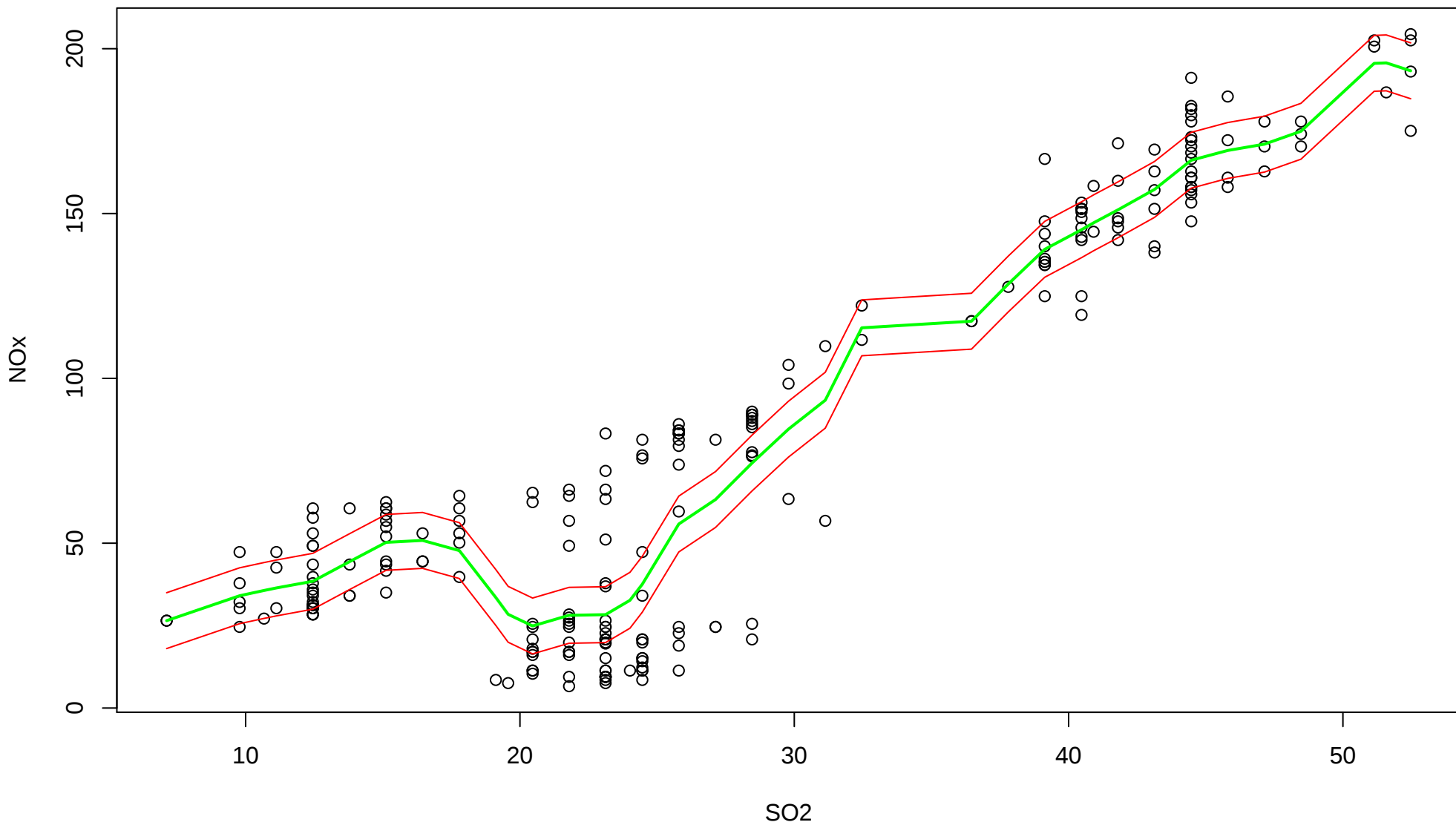
Estimador Local-Linear
