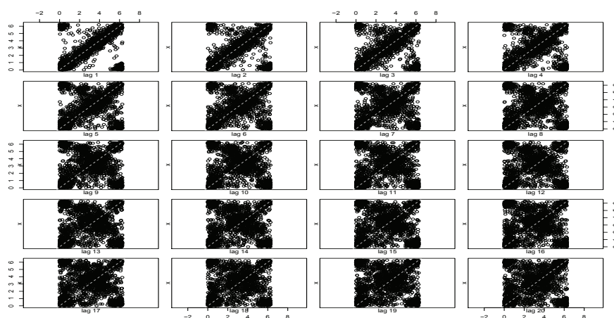
Figura 5.38: Representación de la serie de tiempo de la dirección del viento del tercer periodo de 2010 frente a sus retardos.
