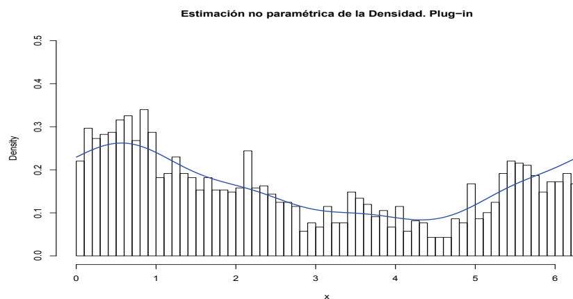
Figura 5.12: Estimación plug-in de la densidad del segundo periodo de 2010
