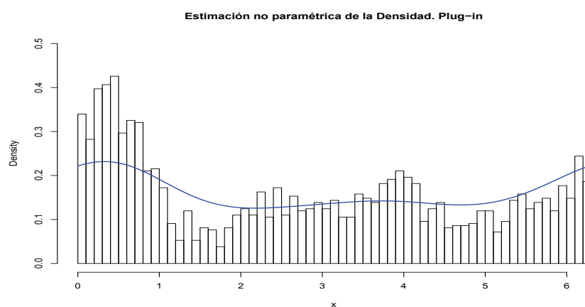
Figura 5.13: Estimación plug-in de la densidad del tercer periodo de 2010
