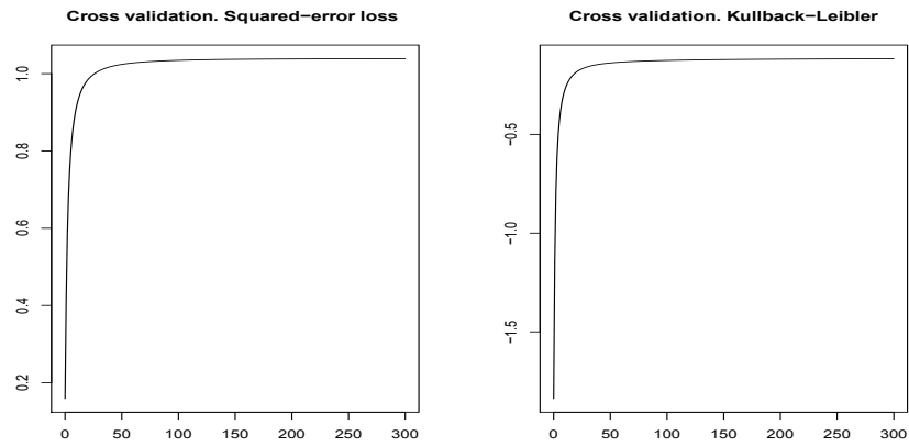
Figura 5.27: Validación cruzada del cuarto periodo de 2010
