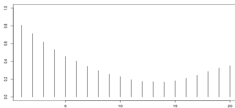
Figura 5.34: Autocorrelaciones circulares de la direcci6n de viento del segundo periodo de 2010
