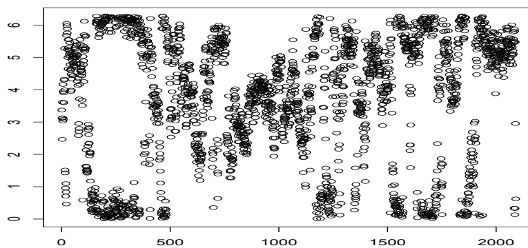
Figura 5.9: Gráfico de dispersión de los datos de dirección de viento del cuarto periodo de 2010
