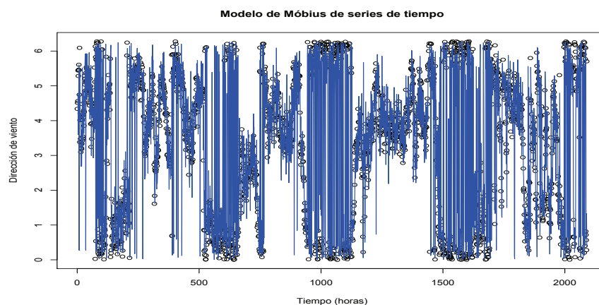
Figura 5.33: Serie de tiempo de la direcci6n de viento del primer periodo de 2010
