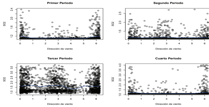
Figura 5.58: Estimación de la función de regresión circular-lineal en F2. Estimación del parámetro de suavizado mediante validación cruzada.
