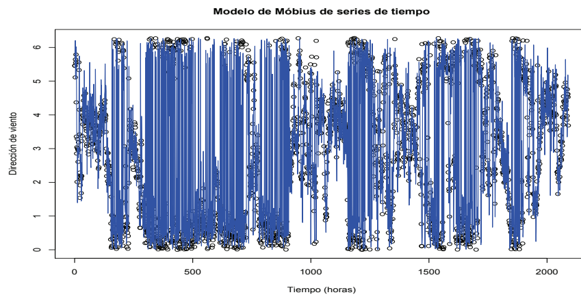
Figura 5.39: Serie de tiempo de la dirección de viento del tercer periodo de 2010
