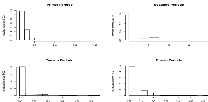
Figura 5.43: Representación del histograma de las medias horarias de SO_2 medido en la estación B1
