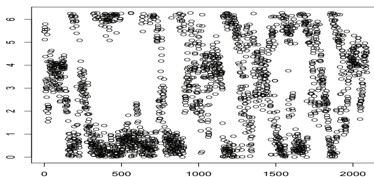
Figura 5.7: Gráfico de dispersión de los datos de dirección de viento del tercer periodo de 2010
