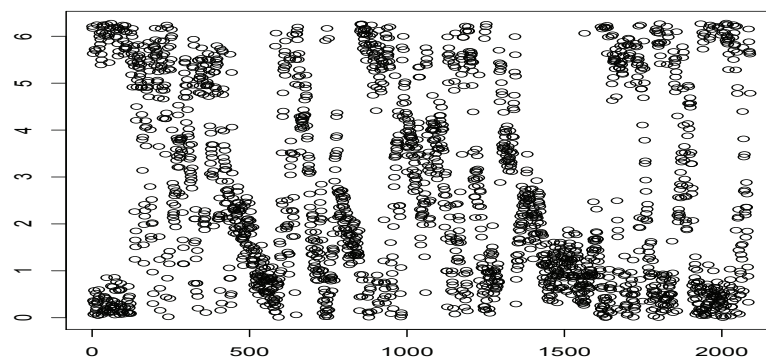
Figura 5.5: Gráfico de dispersión de los datos de dirección de viento del segundo periodo de 2010
