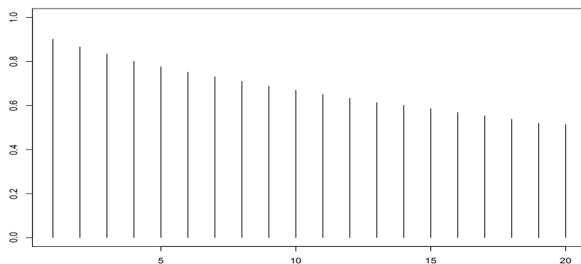
Figura 5.31: Autocorrelaciones circulares para dirección de viento del primer periodo de 2010
