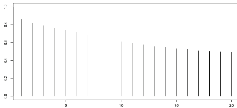
Figura 5.40: Autocorrelaciones circulares de la dirección de viento del cuarto periodo de 2010
