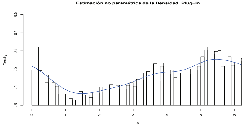
Figura 5.14: Estimación plug-in de la densidad del cuarto periodo de 2010
