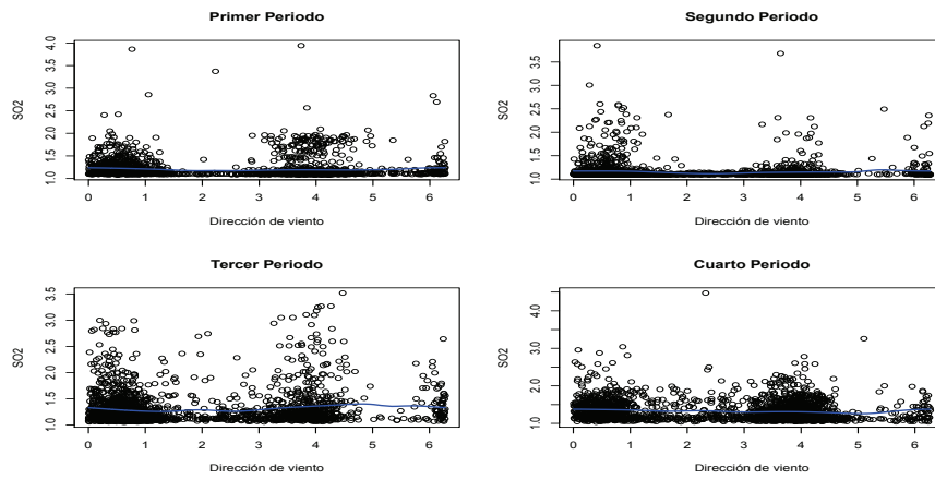
Figura 5.53: Estimación de la función de regresión circular-lineal en B2. Estimación del parámetro de suavizado mediante 1/h_s^2 .
