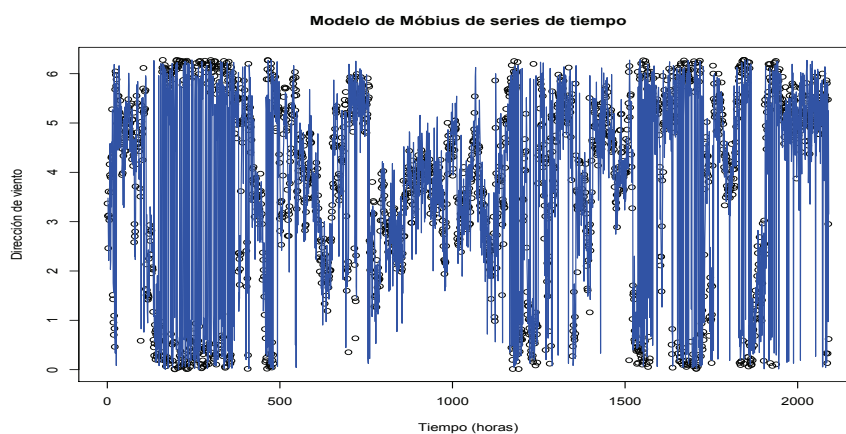
Figura 5.42: Serie de tiempo de la dirección de viento del cuarto periodo de 2010
