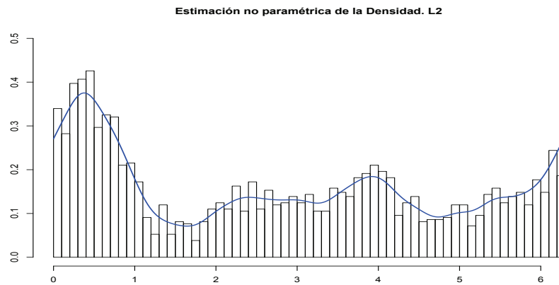
Figura 5.24: Estimación L2 de la densidad del tercer periodo de 2010
