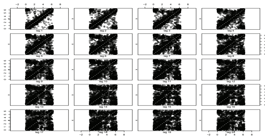
Figura 5.35: Representación de la serie de tiempo de la dirección del viento del segundo periodo de 2010 frente a sus retardos.
