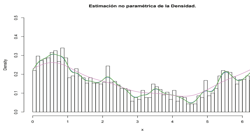
Figura 5.22: Estimación no paramétrica de la Densidad. L2 (azul), KL (verde), plug-in (violeta)
