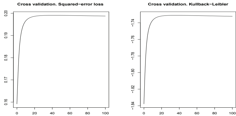
Figura 5.23: Validación cruzada del tercer periodo de 2010
