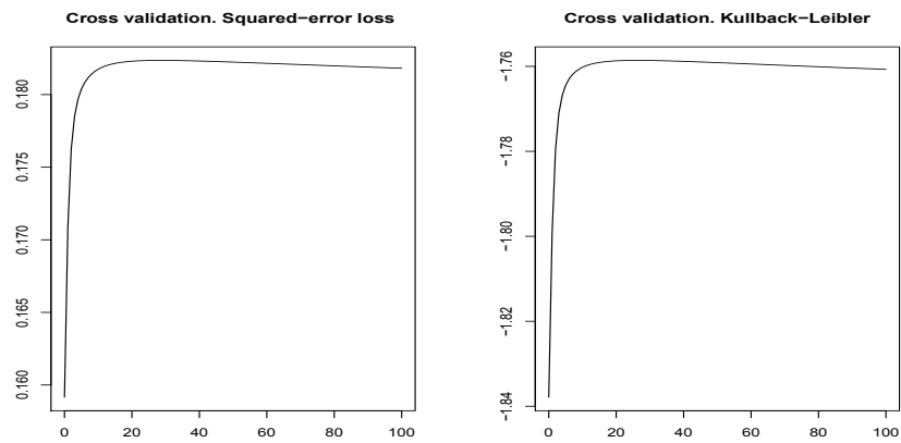
Figura 5.15: Validación cruzada del primer periodo de 2010
