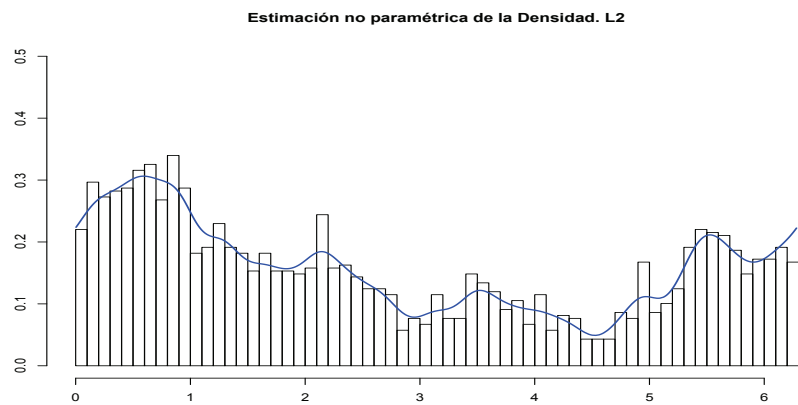
Figura 5.20: Estimación L2 de la densidad del segundo periodo de 2010
