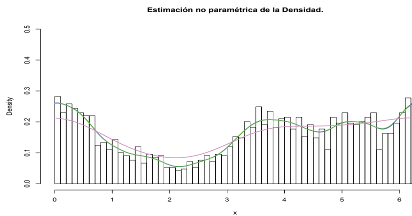
Figura 5.18: Estimación no paramétrica de la Densidad. L2 (azul), KL (verde), plug-in (violeta)
