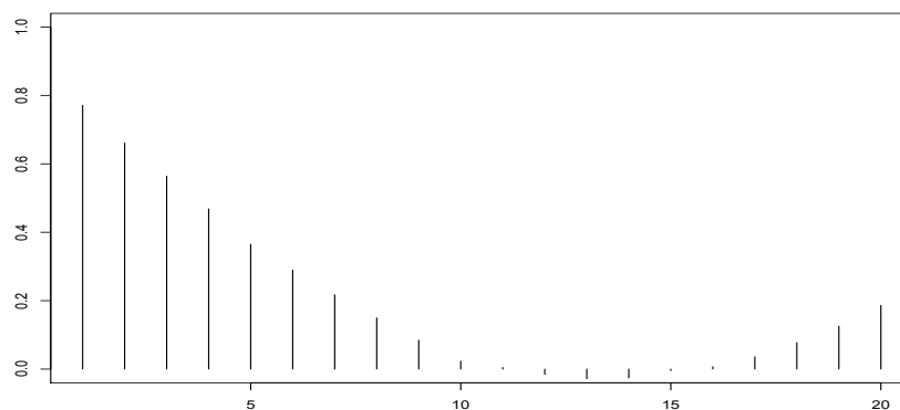
Figura 5.37: Autocorrelaciones circulares de la dirección de viento del tercer periodo de 2010
