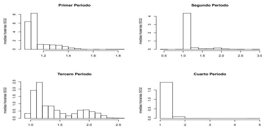
Figura 5.45: Representación del histograma de las medias horarias de SO_2 medido en la estación C9
