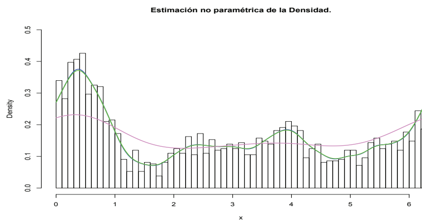
Figura 5.26: Estimación no paramétrica de la Densidad. L2 (azul), KL (verde), plug-in (violeta)
