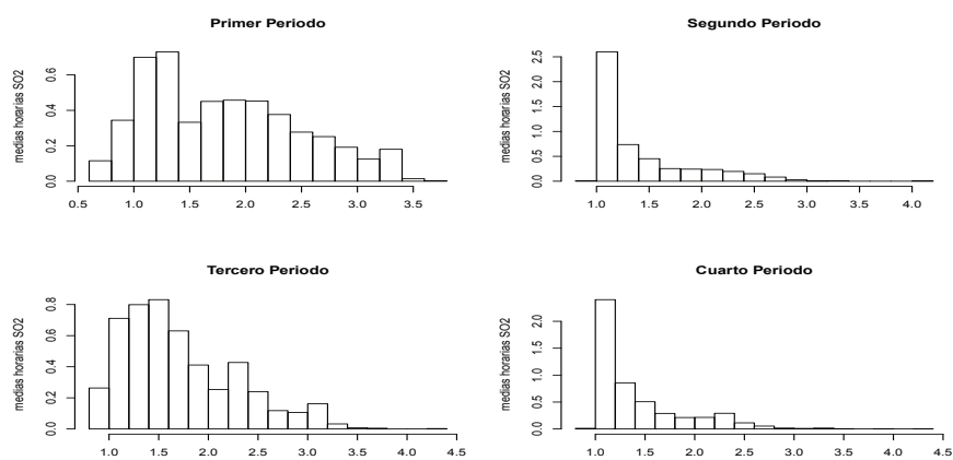
Figura 5.47: Representación del histograma de las medias horarias de SO_2 medido en la estación G2
