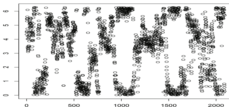
Figura 5.3: Gráfico de dispersión de los datos de dirección de viento del primer periodo de 2010
