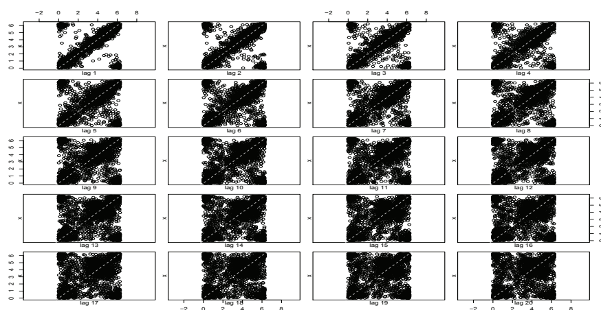
Figura 5.32: Representación de la serie de tiempo de la dirección del viento del primer periodo de 2010 frente a sus retardos.
