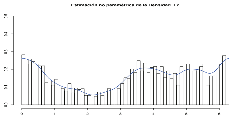
Figura 5.16: Estimación L2 de la densidad del primer periodo de 2010
