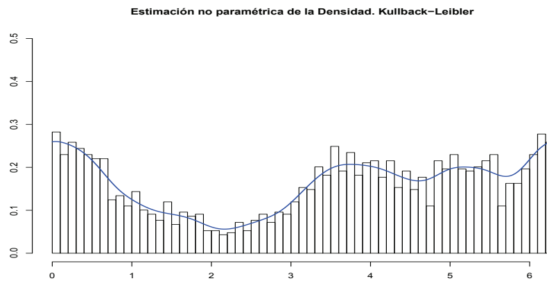
Figura 5.17: Estimación KL de la densidad del primer periodo de 2010
