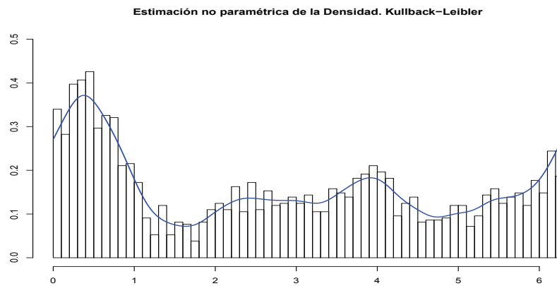
Figura 5.25: Estimación KL de la densidad del tercer periodo de 2010
