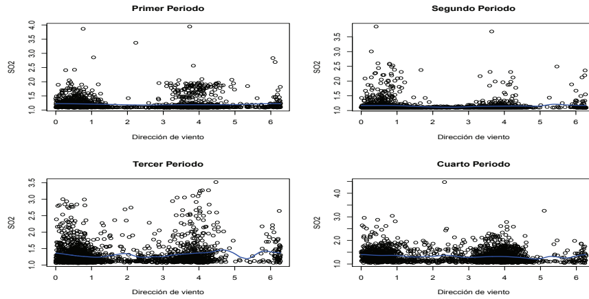
Figura 5.52: Estimación de la función de regresión circular-lineal en B2. Estimación del parámetro de suavizado mediante validación cruzada.
