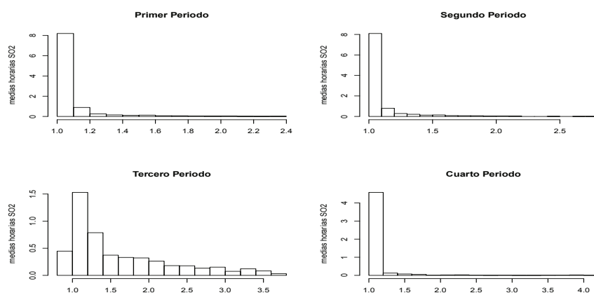
Figura 5.46: Representación del histograma de las medias horarias de SO_2 medido en la estación F2
