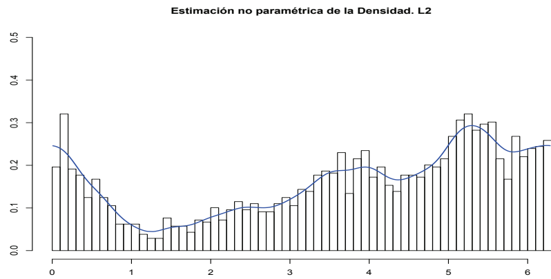
Figura 5.28: Estimación L2 de la densidad del cuarto periodo de 2010
