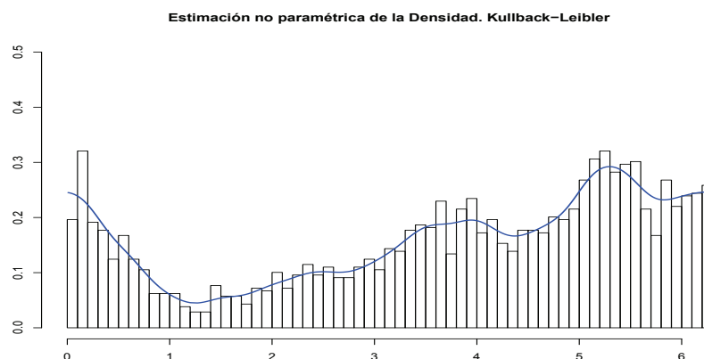
Figura 5.29: Estimación KL de la densidad del cuarto periodo de 2010
