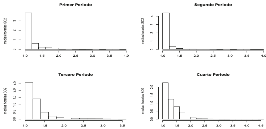
Figura 5.44: Representación del histograma de las medias horarias de SO_2 medido en la estación B2
