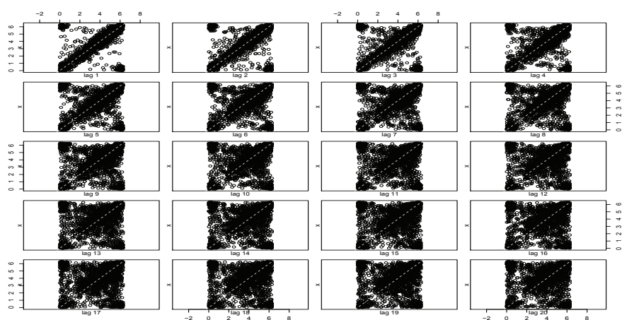
Figura 5.41: Representación de la serie de tiempo de la dirección del viento del cuarto periodo de 2010 frente a sus retardos.
