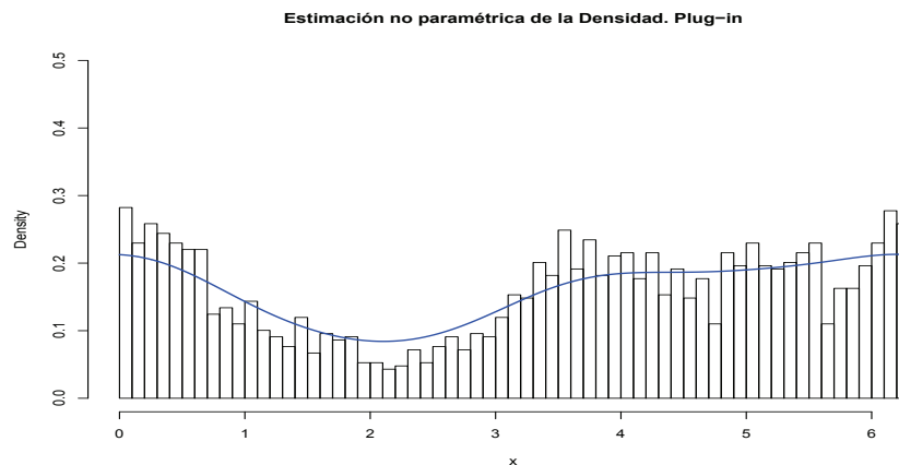
Figura 5.11: Estimación plug-in de la densidad del primer periodo de 2010
