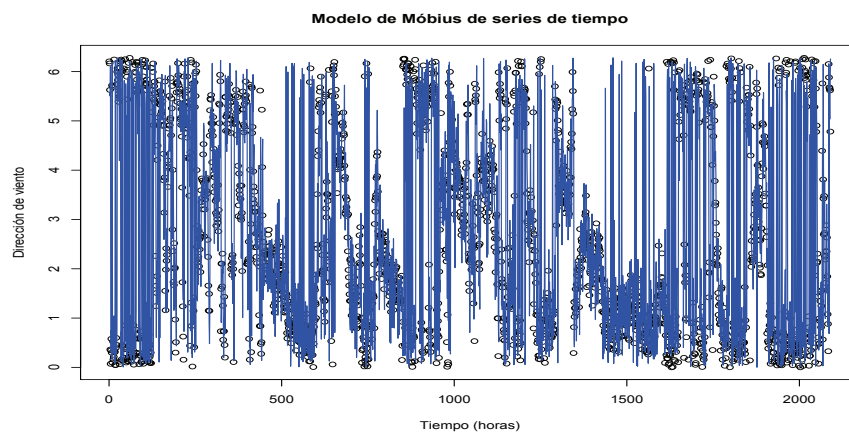
Figura 5.36: Serie de tiempo de la dirección de viento del segundo periodo de 2010
