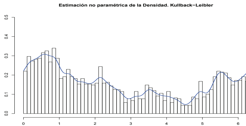
Figura 5.21: Estimación KL de la densidad del segundo periodo de 2010
