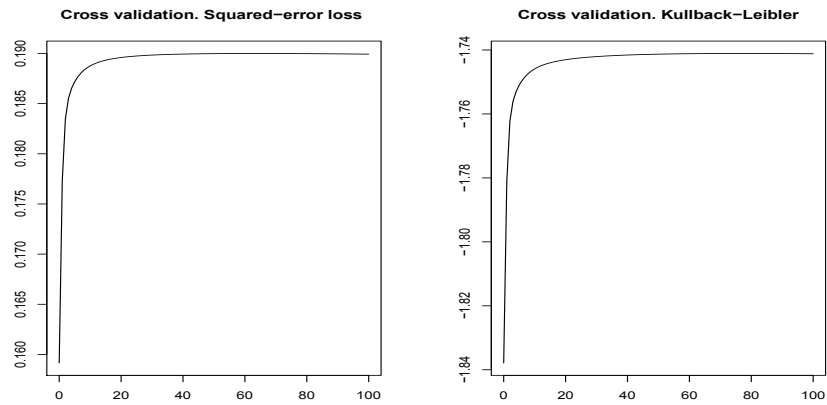
Figura 5.19: Validación cruzada del segundo periodo de 2010
