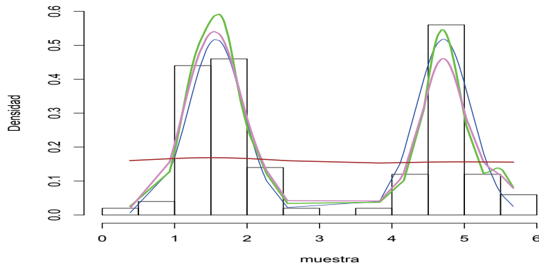
Figura 2.1: Representación de la densidad teórica de una mixtura de von Mises vM(\pi/2,15), vM(3\pi/2,15) y la estimación no paramétrica de la densidad seleccionando el parámetro de suavizado mediante las técnicas estudiadas. L2 (verde), KL (violeta), plug-in (marrón)
