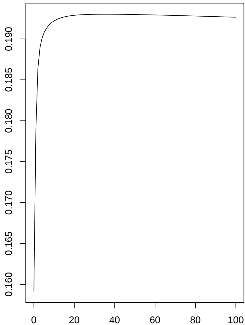
Validación cruzada (L2)
