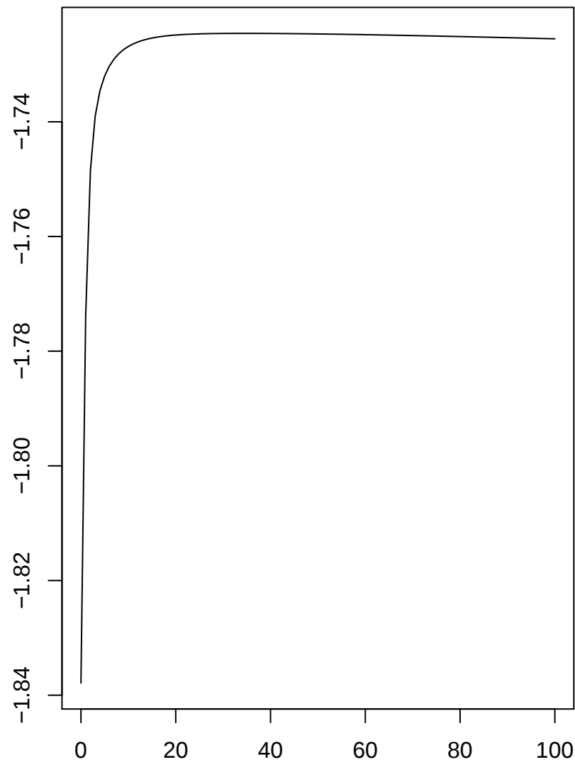
Validación cruzada (Kullback-Leibler)
