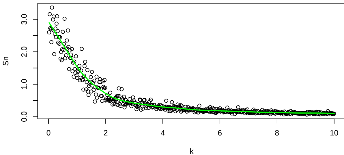
Estimador Local-Linear
