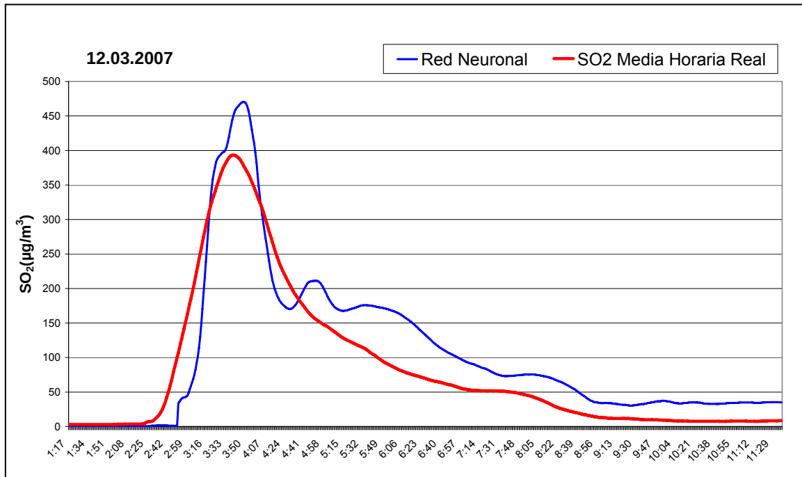
Figura 2.9: Episodio de alteración de la calidad del aire ocurrido en el 12 de Marzo de 2003. Predicción dada por red neuronal
