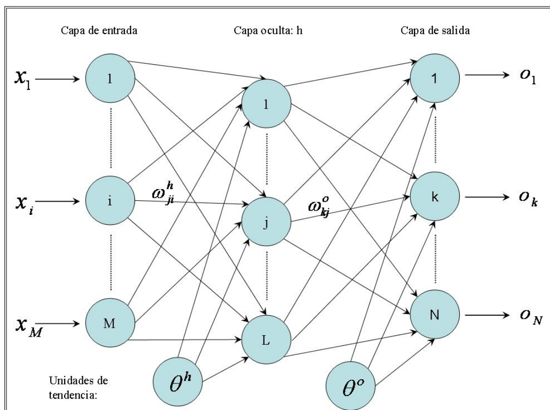
Figura 2.6: Esquema general de una red neuronal multicapa (MLP).
