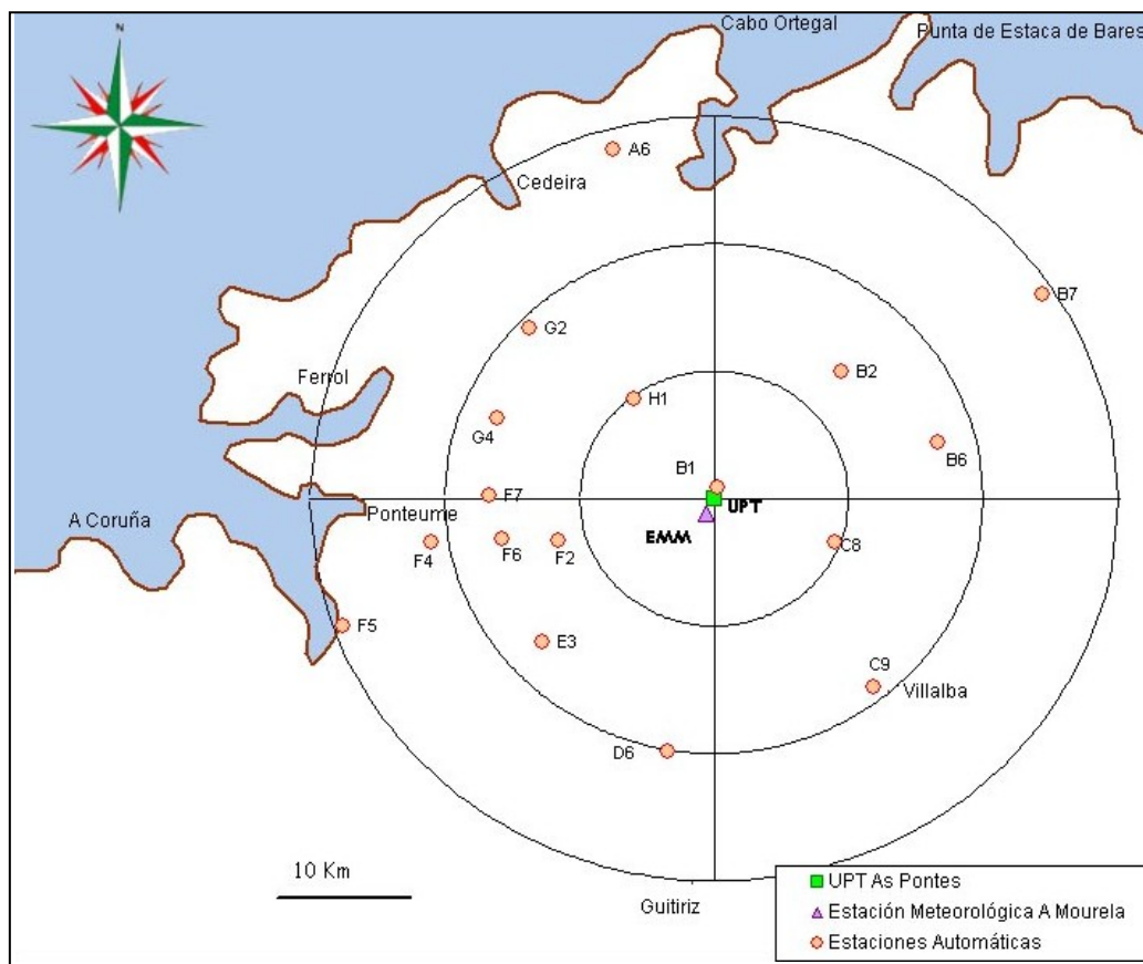
Figura 1.1: Red de Vigilancia y Control de la Calidad Atmosférica de la Central Térmica de As Pontes, propiedad de Endesa Generación S. A. (Noroeste de España)
