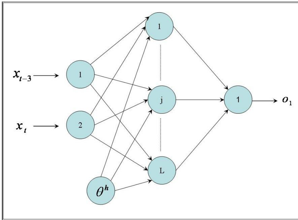
Figura 2.7: Esquema de una red neuronal diseñada para predecir el nivel de emisión de \text{SO}_2 en media horaria, con media hora de antelación.
