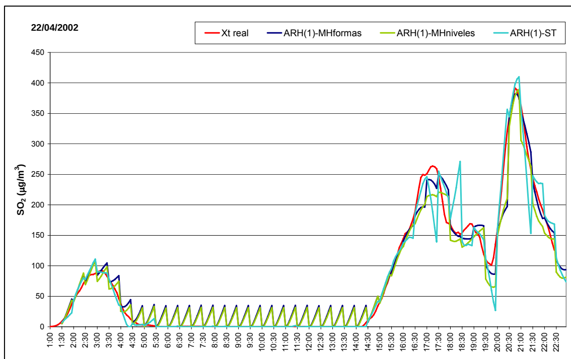
Figura 2.13: Episodio correspondiente al día 22 de abril de 2002. Predicciones de ARH(1), utilizando matriz histórica de formas, de niveles y sin matriz histórica (ST) (Fernández de Castro, et al., 2005).
