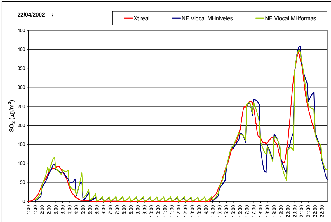
Figura 2.11: Episodio correspondiente al día 22 de abril de 2002. Predicciones de Núcleo Funcional con ventana local, utilizando matriz histórica de niveles y de formas (Fernández de Castro, et al., 2005).
