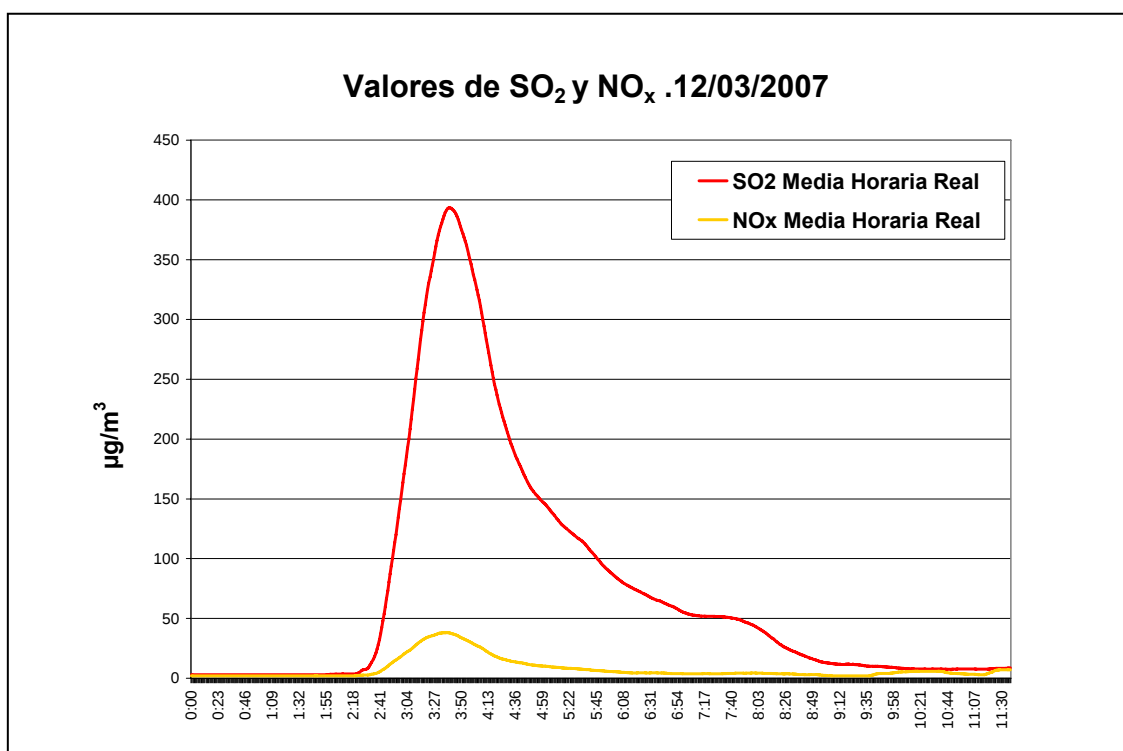
Figura 1.3: Episodio de alteración de la calidad del aire ocurrido en una de las estaciones de medida el 12 de marzo de 2007.
