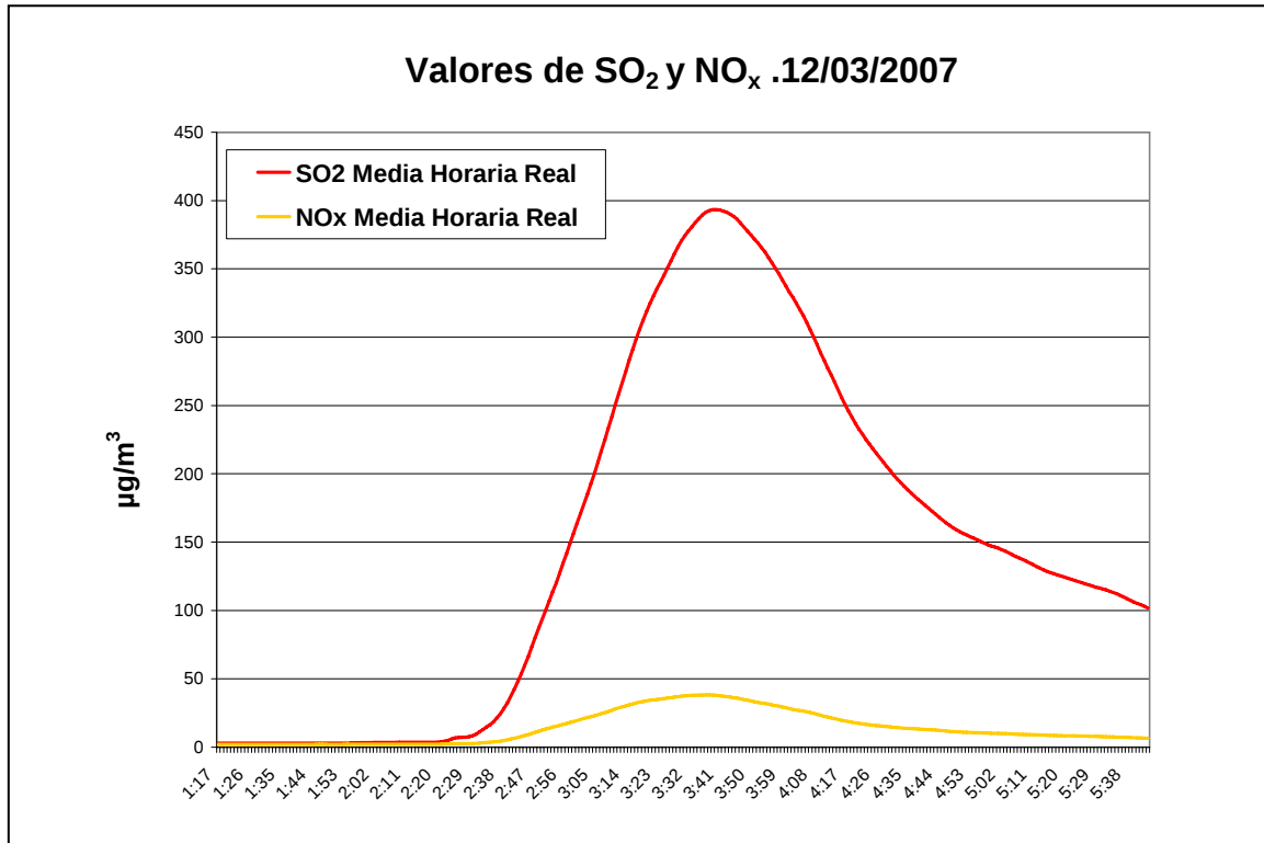
Figura 3.5: Episodio de alteración de la calidad del aire ocurrido el 12 de Marzo de 2007.
