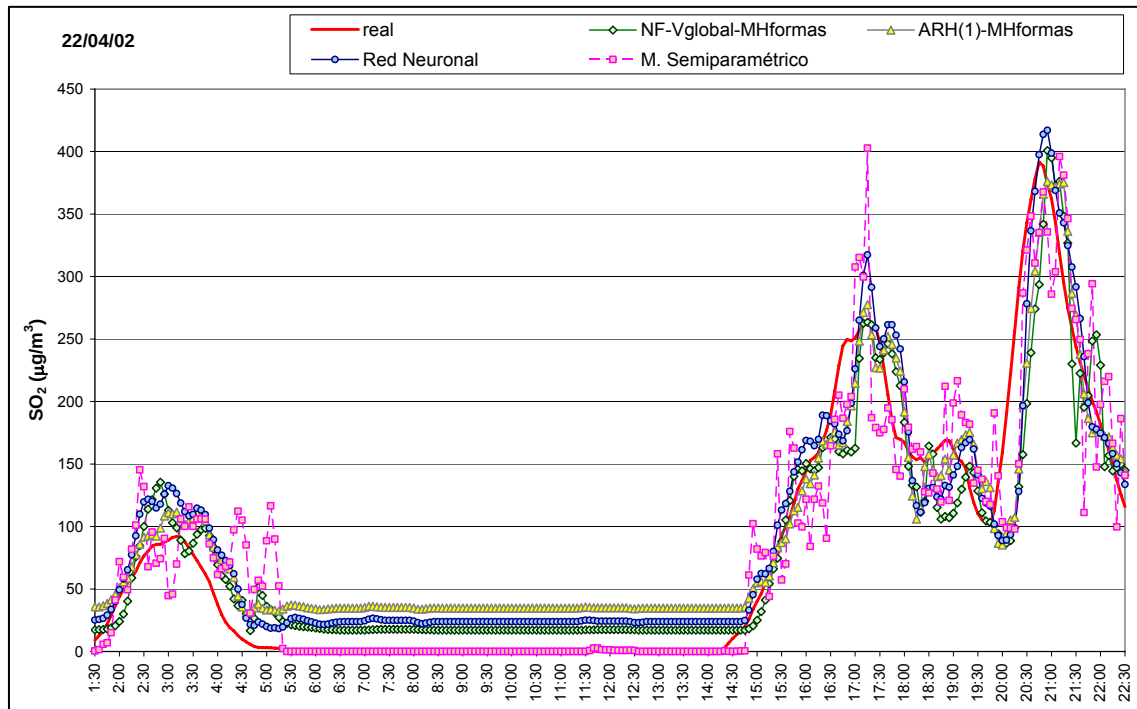
Figura 2.14: Episodio correspondiente al día 22 de abril de 2002. Comparación de predicciones de modelos funcionales: ARH(1) y Núcleo Funcional con ventana global, ambos con matriz histórica de formas, y modelos reales: red neuronal y modelo semiparamétrico (Fernández de Castro, et al., 2004).
