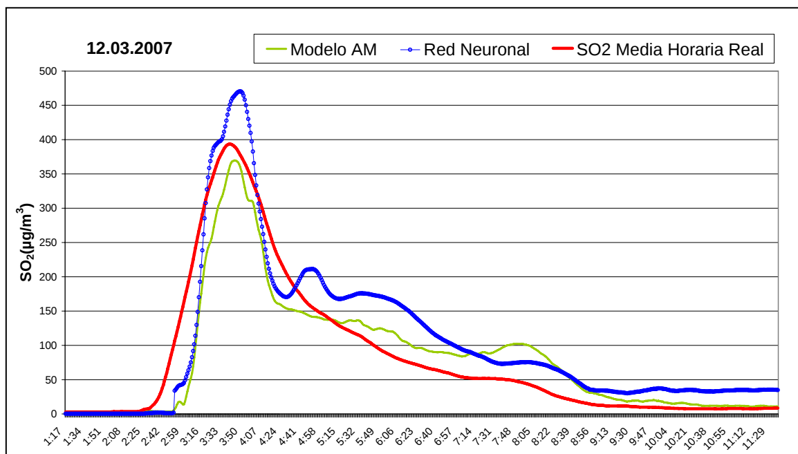
Figura 3.4: Episodio de alteración de la calidad del aire ocurrido el 12 de Marzo de 2007. Predicciones dadas por modelo aditivo y por la Red Neuronal.
