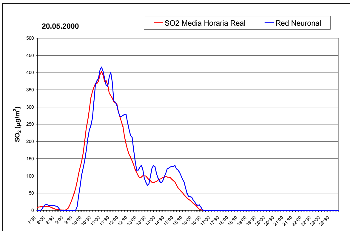
Figura 2.8: Episodio de alteración de la calidad del aire ocurrido el 20 de Mayo de 2000. Predicción dada por red neuronal (Fernández de Castro, et al., 2003).
