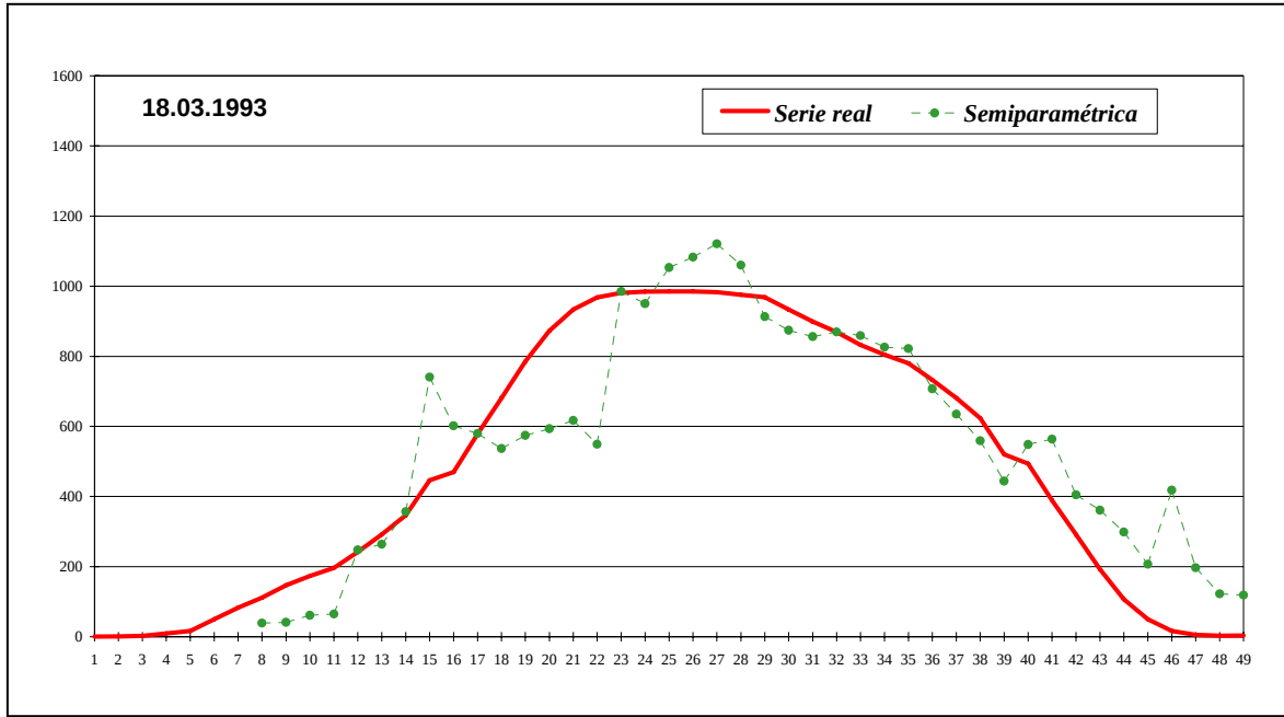
Figura 2.3: Episodio de alteración de la calidad del aire ocurrido en una de las estaciones de medida el 18 de Marzo de 1993. Predicción dada por la metodología semiparamétrica (Prada-Sánchez JM, 1997).
