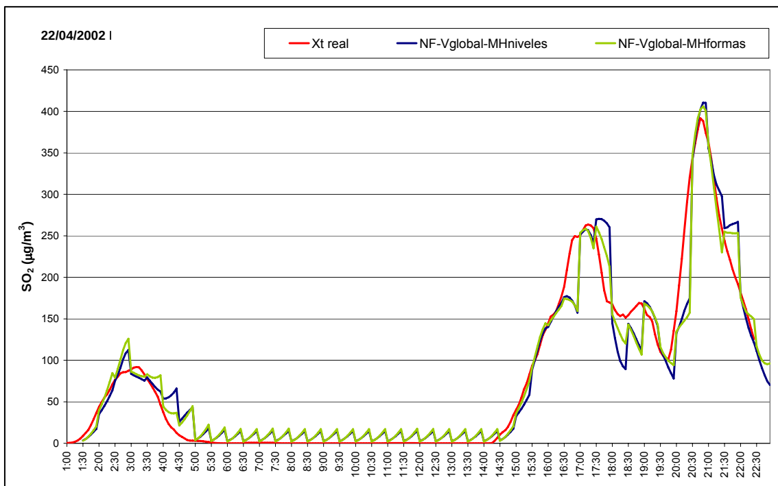
Figura 2.12: Episodio correspondiente al día 22 de abril de 2002. Predicciones de Núcleo Funcional con ventana global, utilizando matriz histórica de niveles y de formas (Fernández de Castro, et al., 2005).
