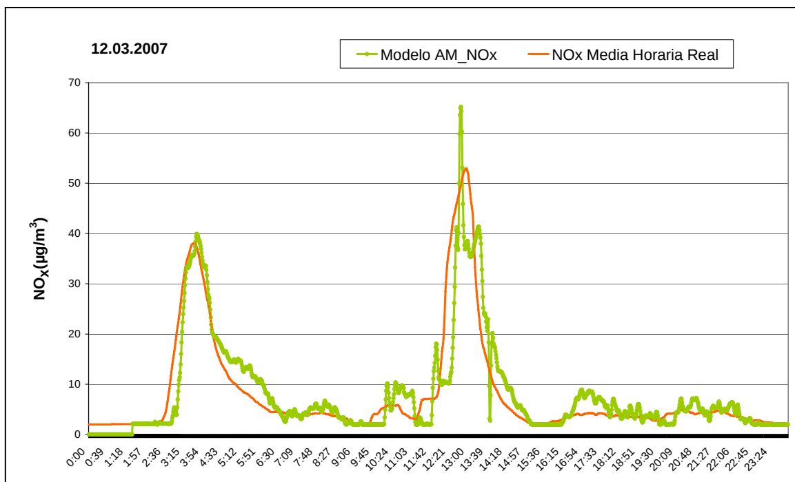
Figura 3.3: Episodio de alteración de la calidad del aire ocurrido el 12 de Marzo de 2007. Predicción dada por modelo aditivo.
