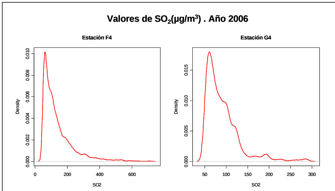
Figura 3.1: Estimación de la densidad de los datos reales de \text{SO}_2 (medidos en \mu\text{g}/\text{m}^3 ) registrados en 2006 para las estaciones F4 y G4.
