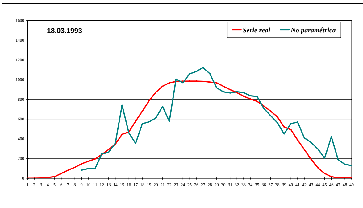
Figura 2.2: Episodio de alteración de la calidad del aire ocurrido en una de las estaciones de medida el 18 de Marzo de 1993. Predicción dada por la metodología no paramétrica (Prada-Sánchez JM, 1997).
