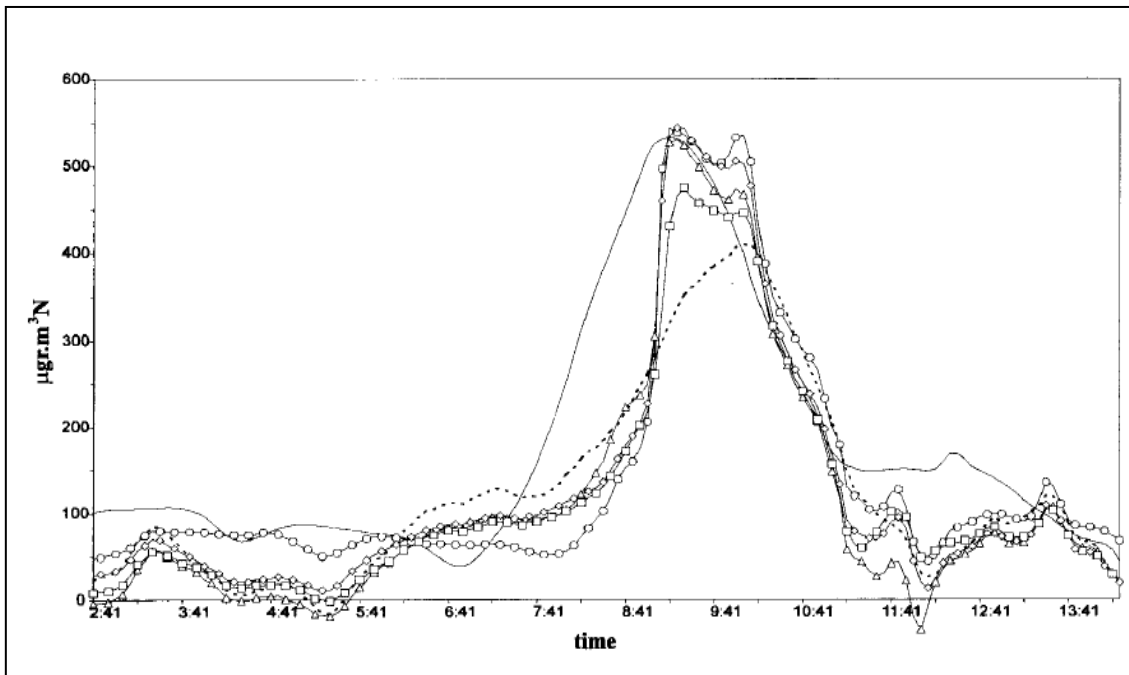
Figura 2.4: Episodio de alteración de la calidad del aire ocurrido el 23 de Agosto 1995 (-). Predicciones dadas por los predictores de ecuaciones (2.2) (círculos), (2.5) (línea discontinua), (2.7) (triángulos), (2.9) (cuadrados) y (2.11) (rombos). Todos ellos utilizan el vector de variables exógenas V^1 (Prada-Sánchez, et. al. , 2000).
