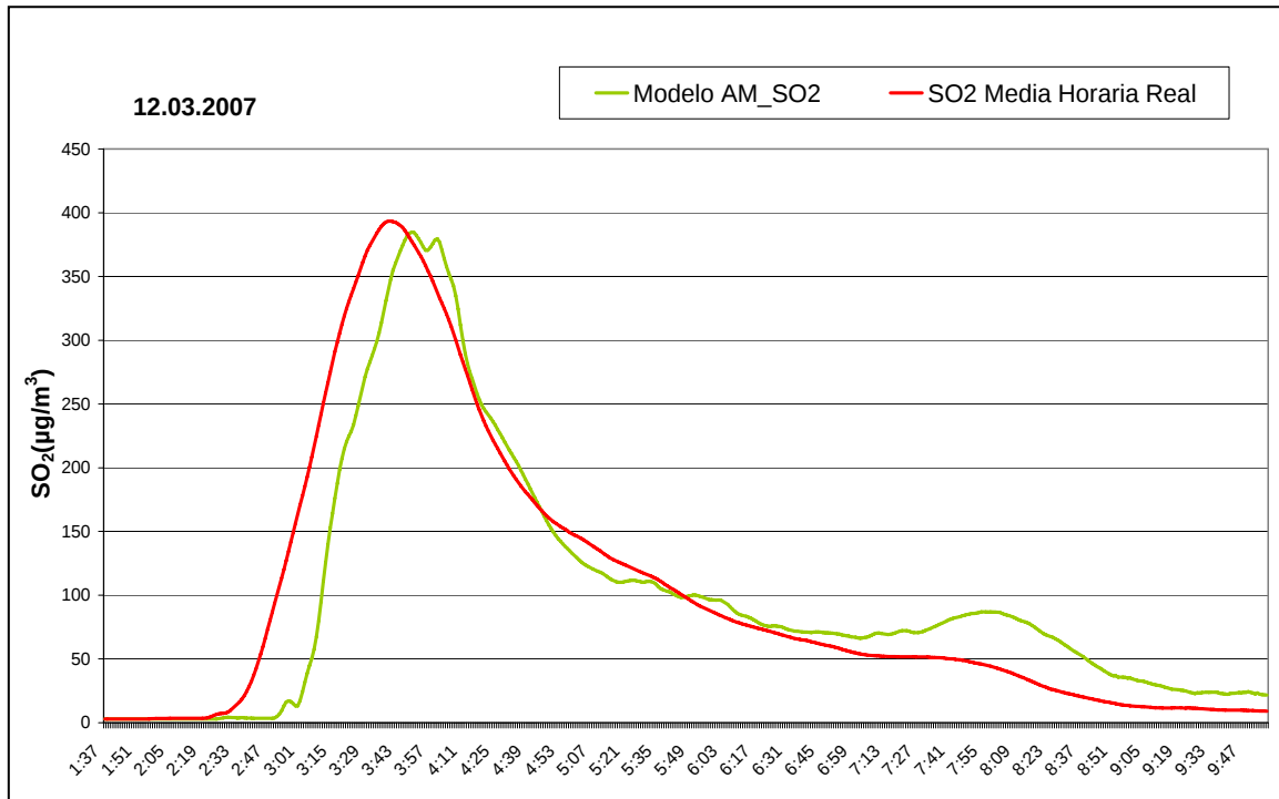
Figura 3.2: Episodio de alteración de la calidad del aire ocurrido el 12 de Marzo de 2007. Predicción dada por modelo aditivo.
