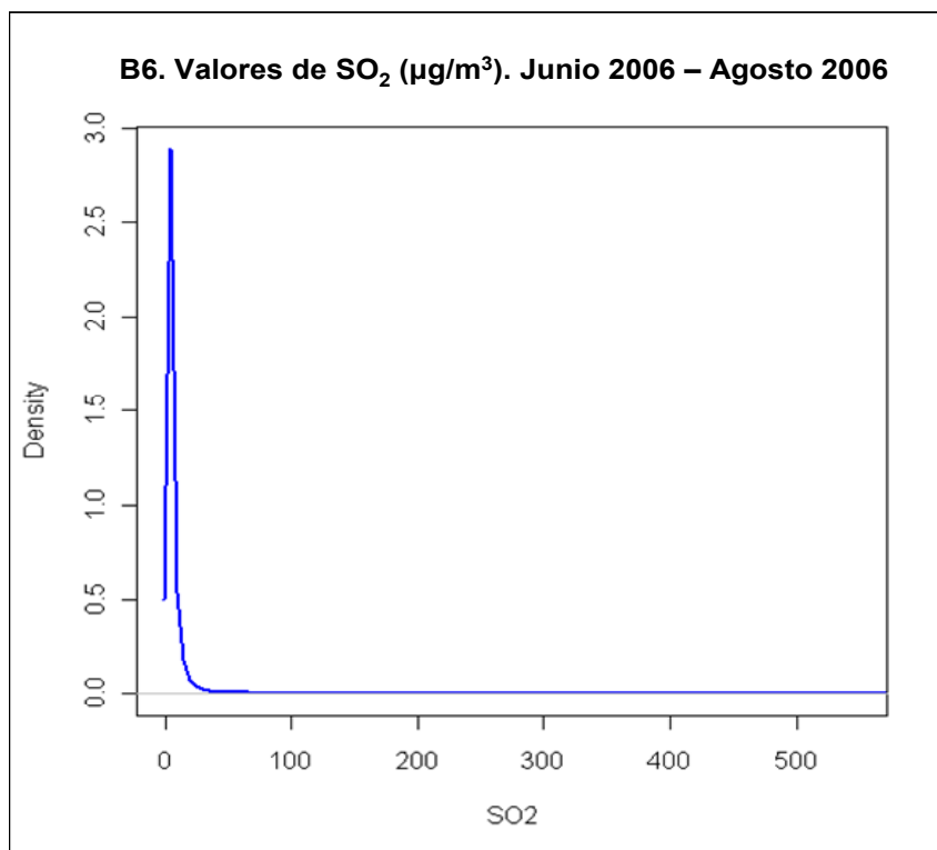
Figura 1.2: Estimación de la densidad de los valores medios horarios de \text{SO}_2 . Estación B6. Período: Junio 2006–Agosto 2006
