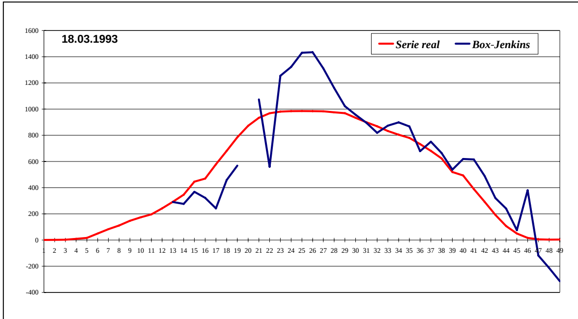
Figura 2.1: Episodio de alteración de la calidad del aire ocurrido en una de las estaciones de medida el 18 de Marzo de 1993. Predicción dada por la metodología Box-Jenkins (Prada-Sánchez, 1997).
