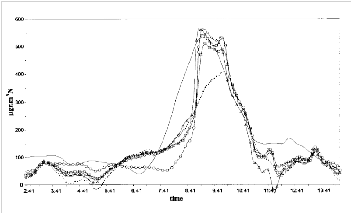
Figura 2.5: Episodio de alteración de la calidad del aire ocurrido el 23 de Agosto 1993. Predicciones dadas por los predictores de ecuaciones (2.2), (2.5), (2.7), (2.9) y (2.11). Todos ellos utilizan el vector de variables exógenas V^2 (Prada-Sánchez, et. al. , 2000).
